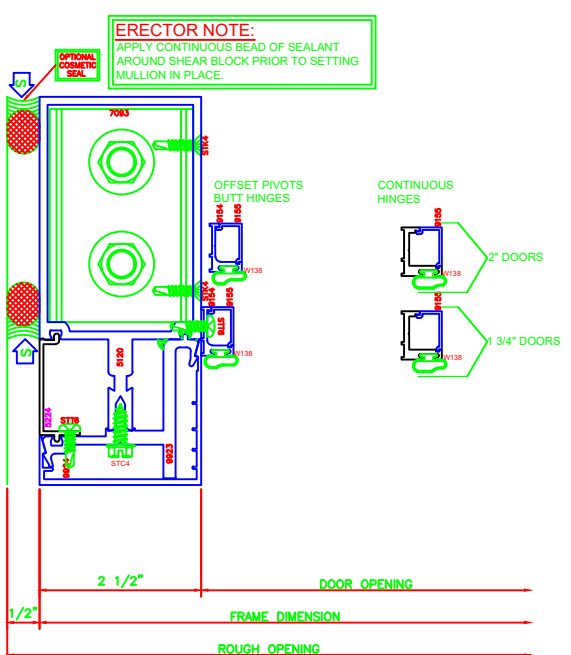
822 O.G. JAMB 5600 6"
