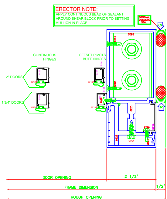
823 O.G. JAMB 5600 6"
